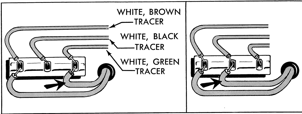
Fig. 2-2 (b). Fan connection for 220-248 volt input.
